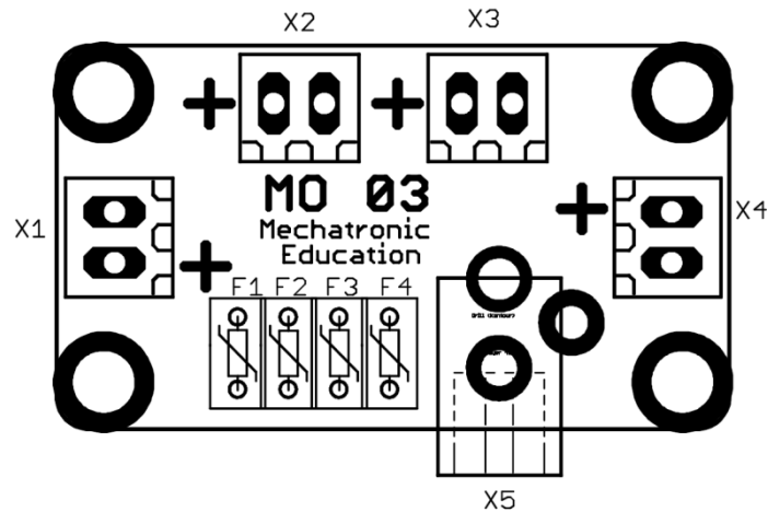
Obrázok 1: Modul MO03
